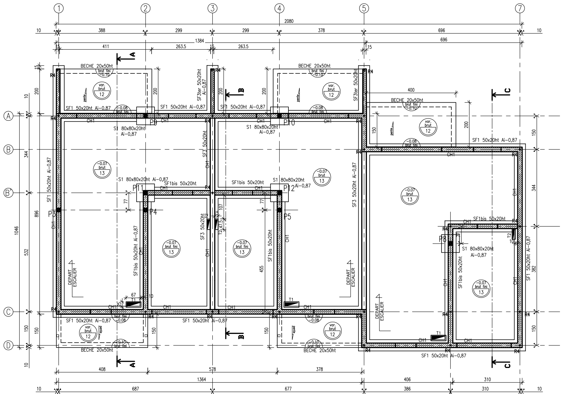
HAMEAU DE PIERRE ILOT G - I PLAN DE FONDATIONS Echelle: 1/100 Cotations en cm
