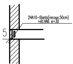
Coupe type
